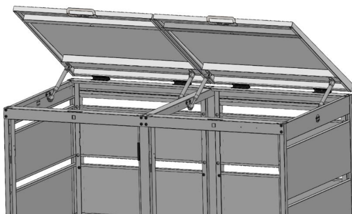
Przykręcenie siłowników i mocowań siłowników Screwing of actuators and actuator mounts
