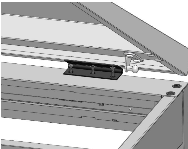
Przykręcenie siłowników i mocowań siłowników Screwing of actuators and actuator mounts
